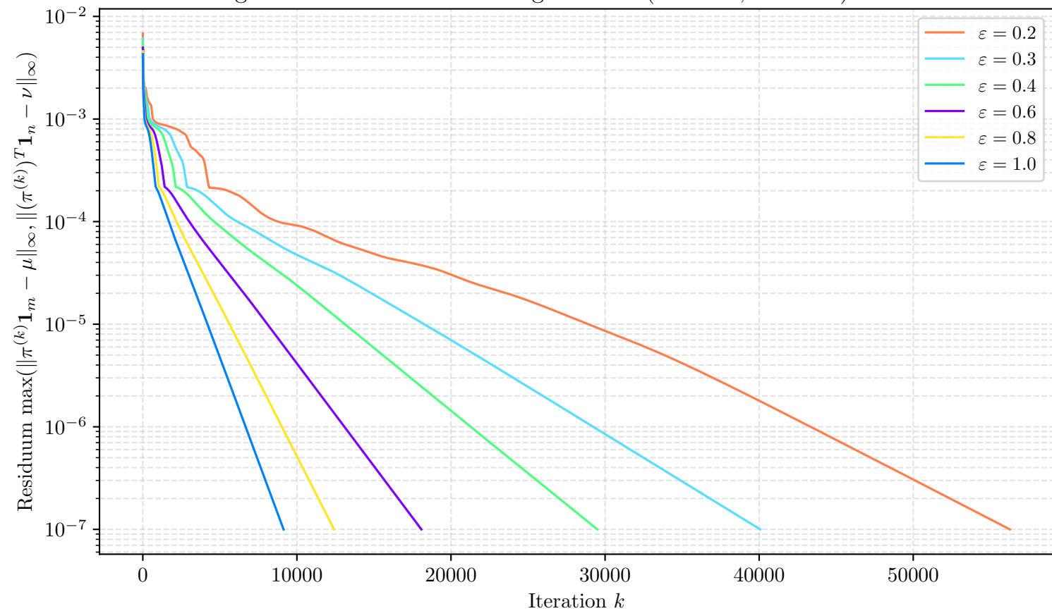
Konvergenzverlauf des Sinkhorn-Algorithmus ( n = 256, m = 256 ) mit Seed=97
