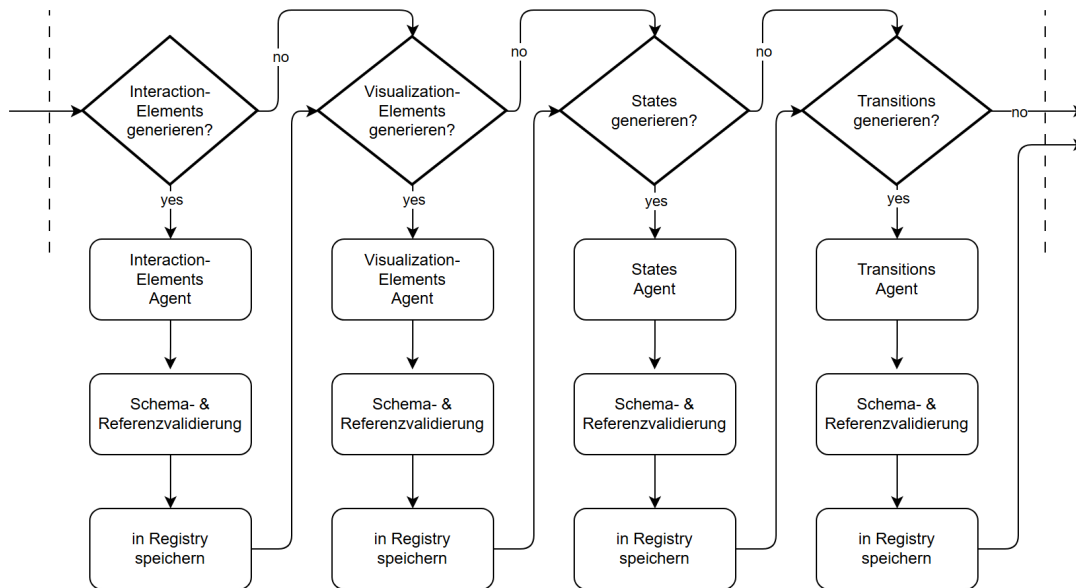
Abbildung 5.6: Specification Generator
