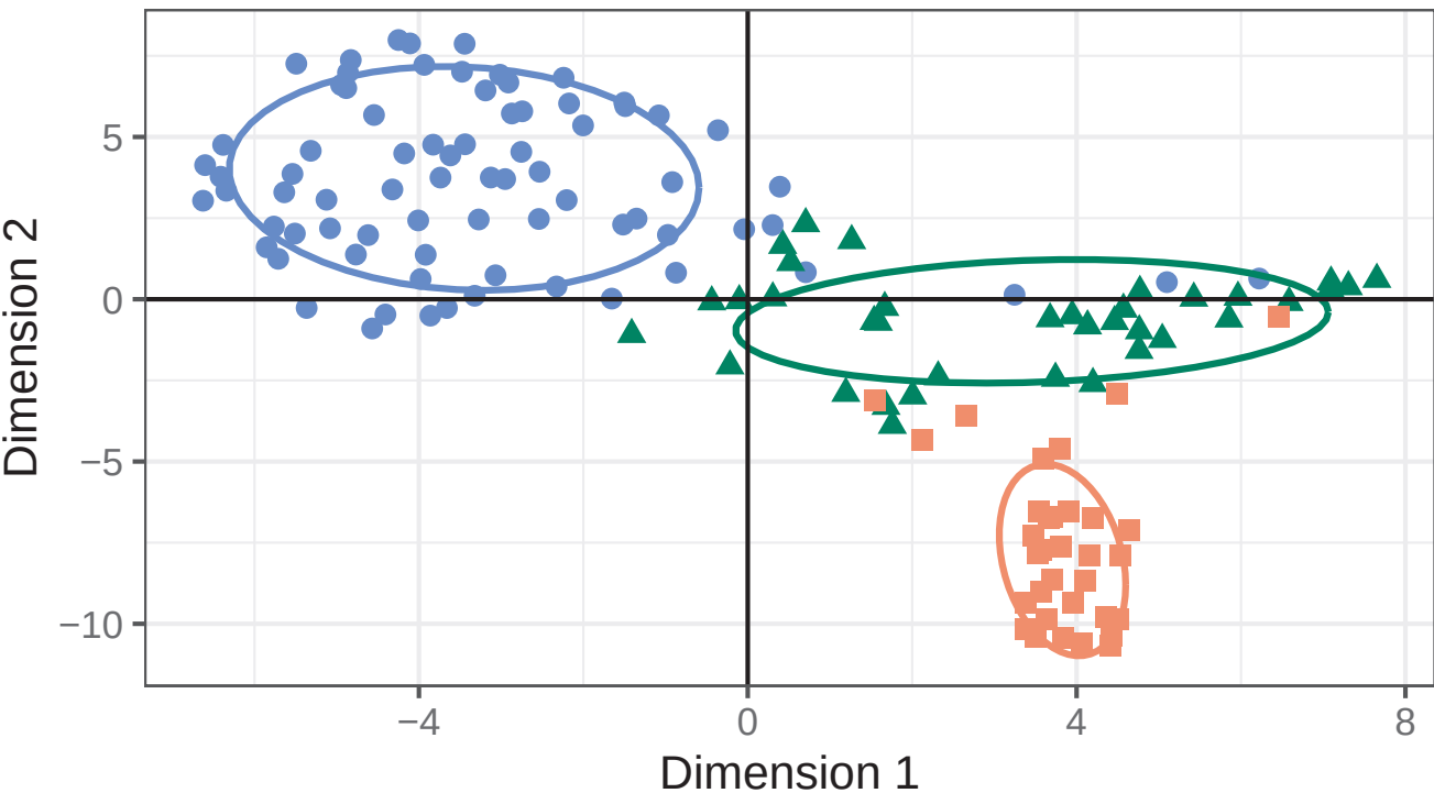
tSNE
