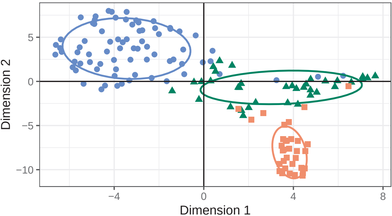
tSNE
