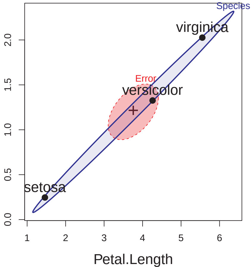
Petal.Width
