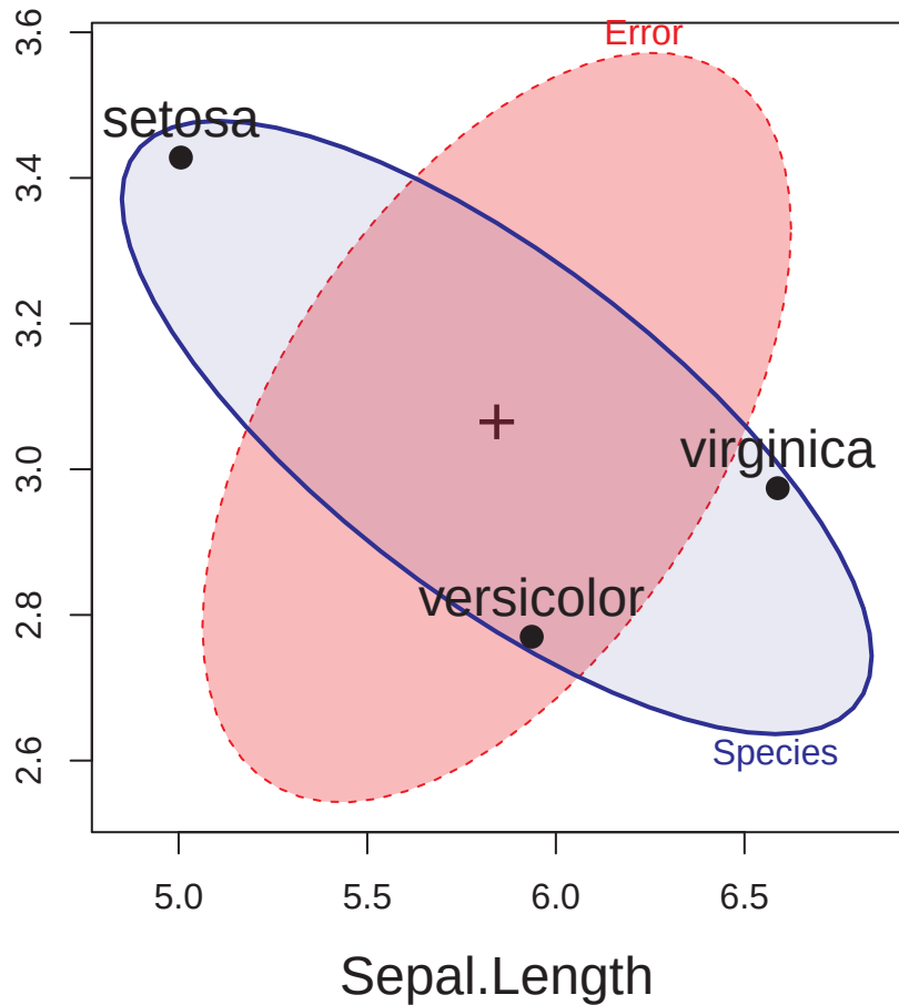
Sepal.Width
