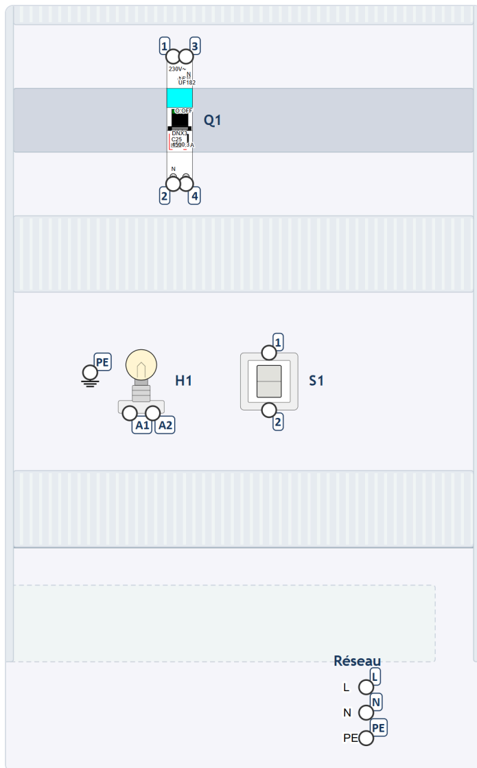
Plan d'implantation
