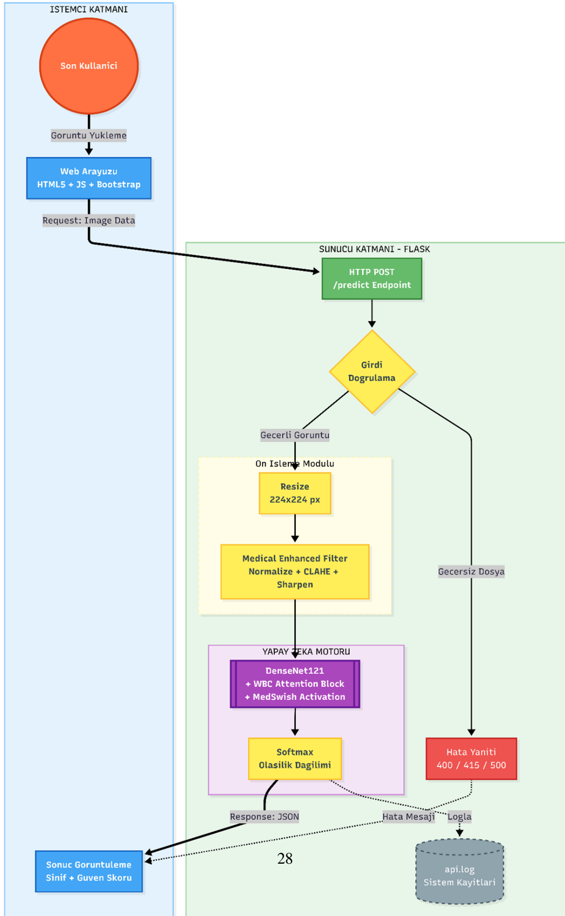
Şekil 8: Sistem Akış Şeması
