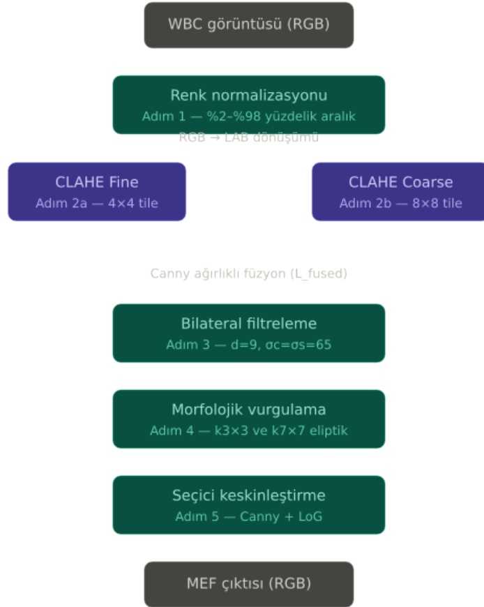
Şekil 4: Preprocess Akış Diyagramı
