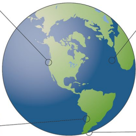
Fermi
