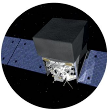
Fermi
