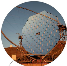
MAGIC
