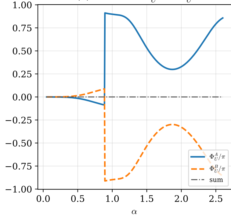
(c) crossed: \Phi_U^B = -\Phi_U^A
