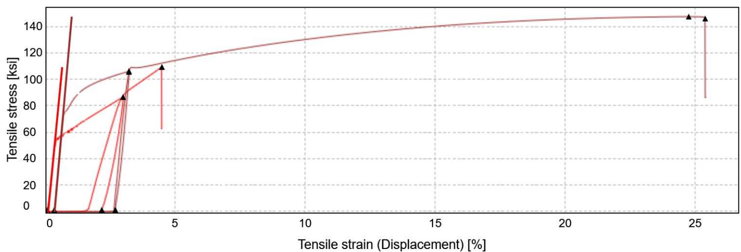
Tensile Test
