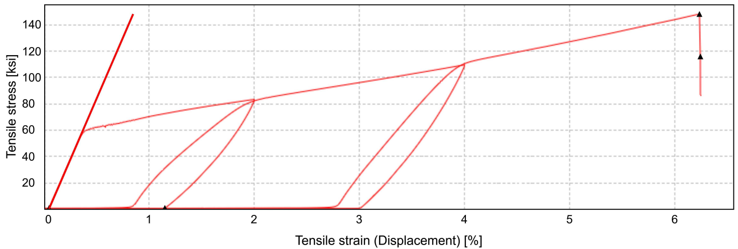
Tensile Test
