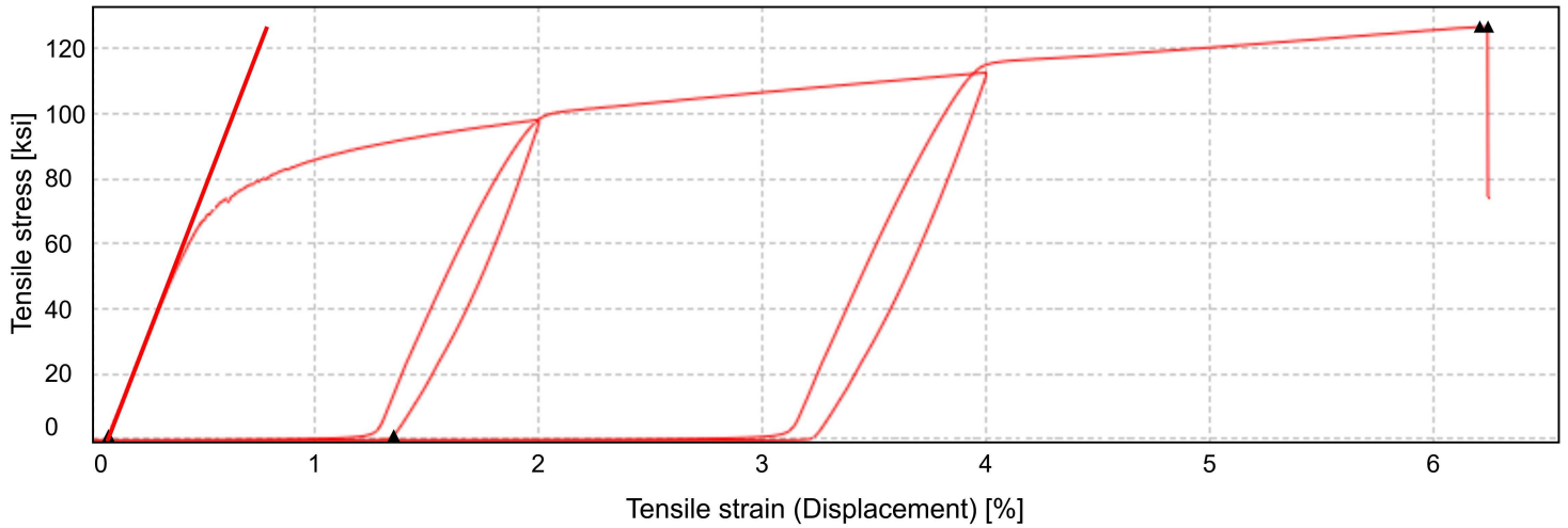
Tensile Test
