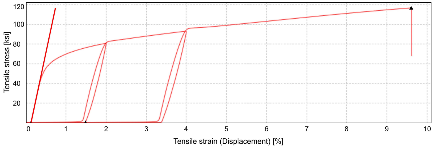
Tensile Test
