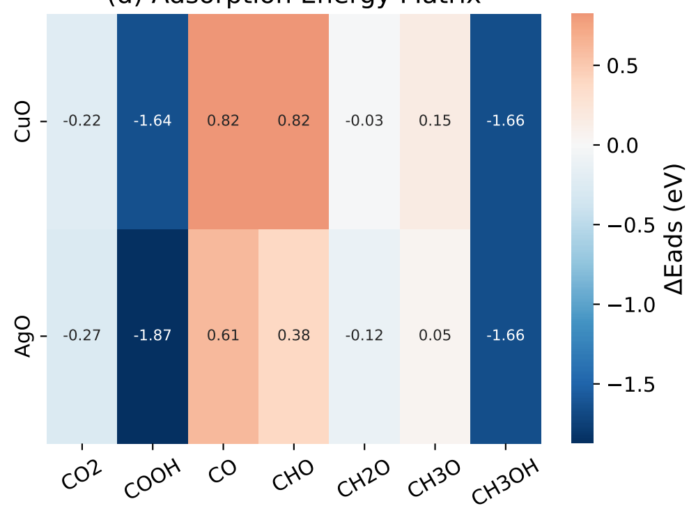
(d) Adsorption Energy Matrix
