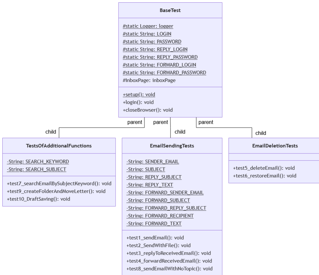
Рисунок 32 – UML-диаграмма пакета Tests
