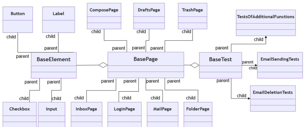
Рисунок 35 – Общая диаграмма классов
