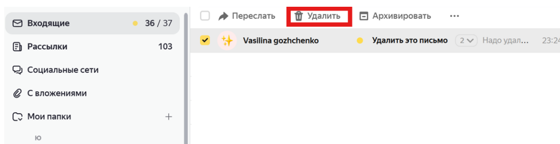
Рисунок 11 – Удаление письма
