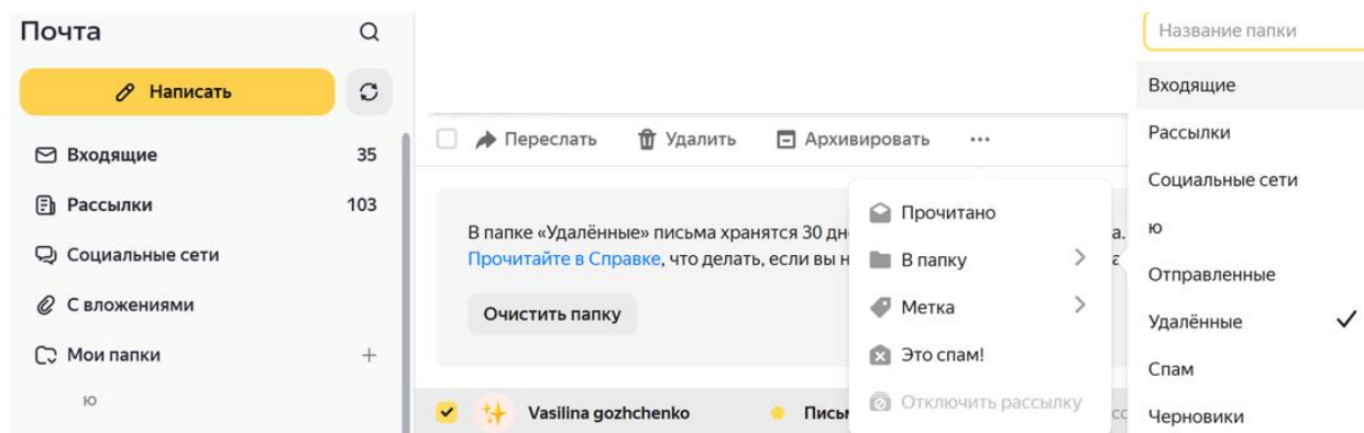
Рисунок 13 – Восстановление письма
