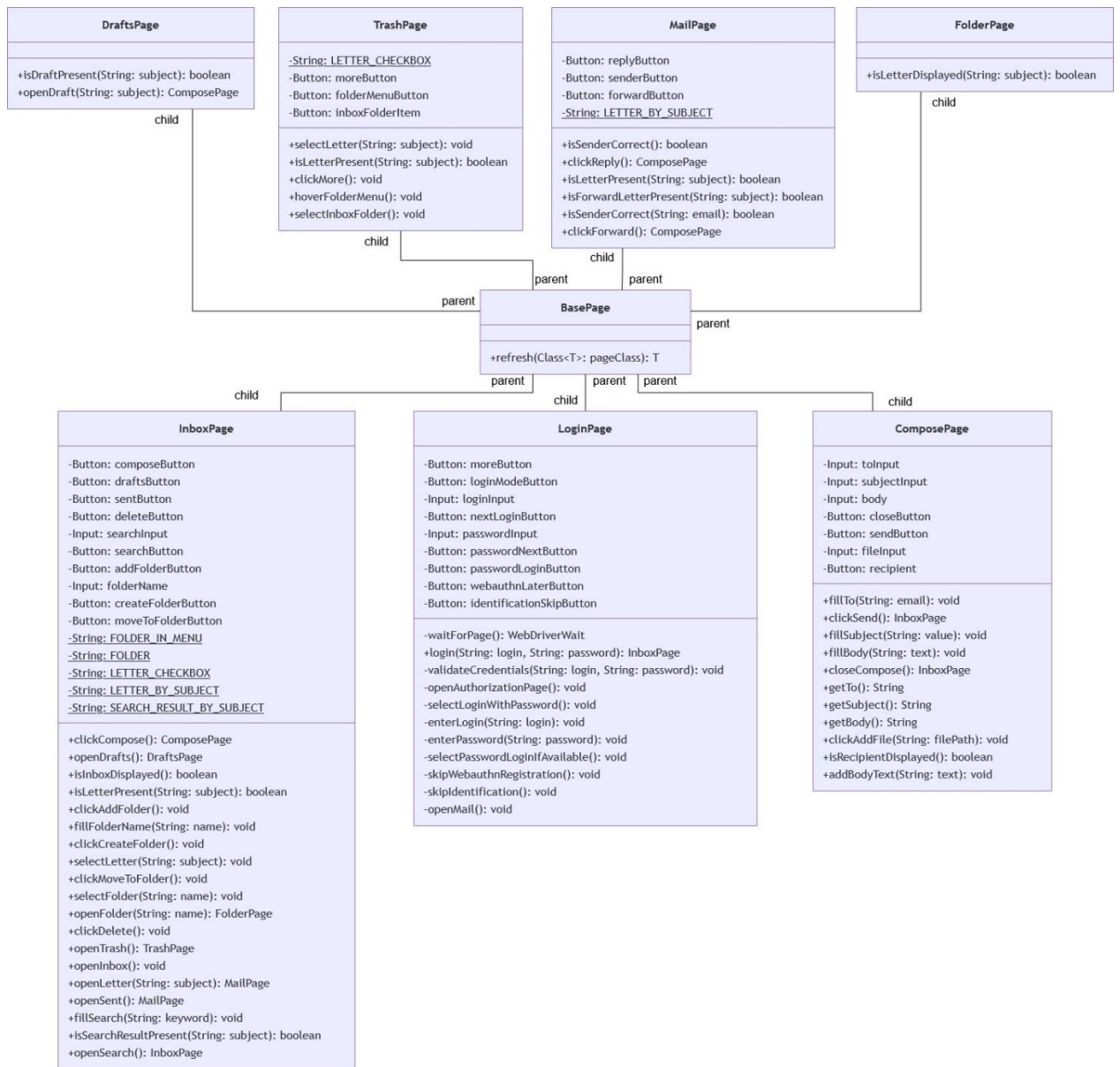
Рисунок 34 – UML-диаграмма пакета Pages
