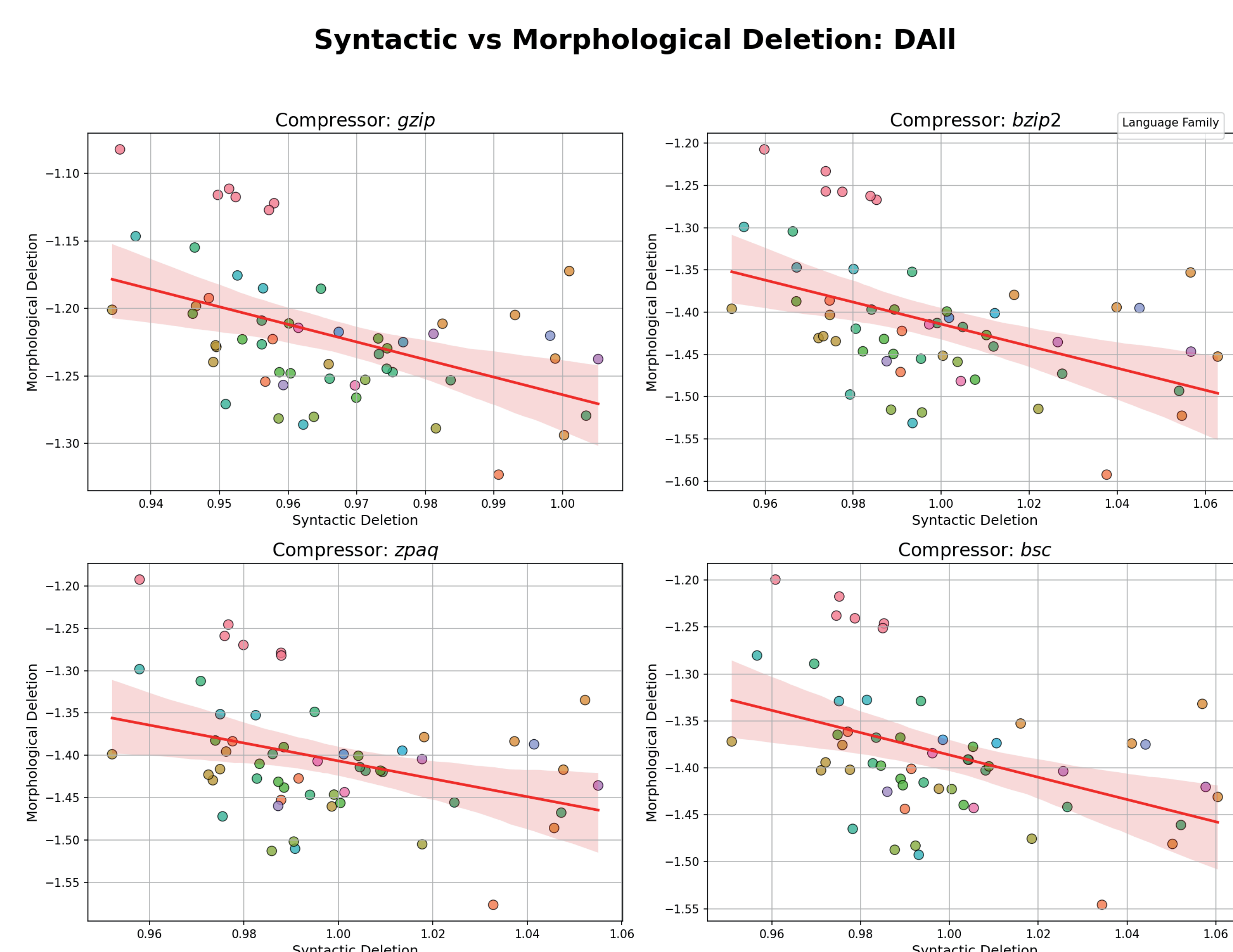
FIGURA 1: GRÁFICO DO SUBCONJUNTO DALL COMPARANDO A COMPLEXIDADE MORFOLÓGICA COM SINTÁTICA PARA DIFERENTES COMPRESSORES.
