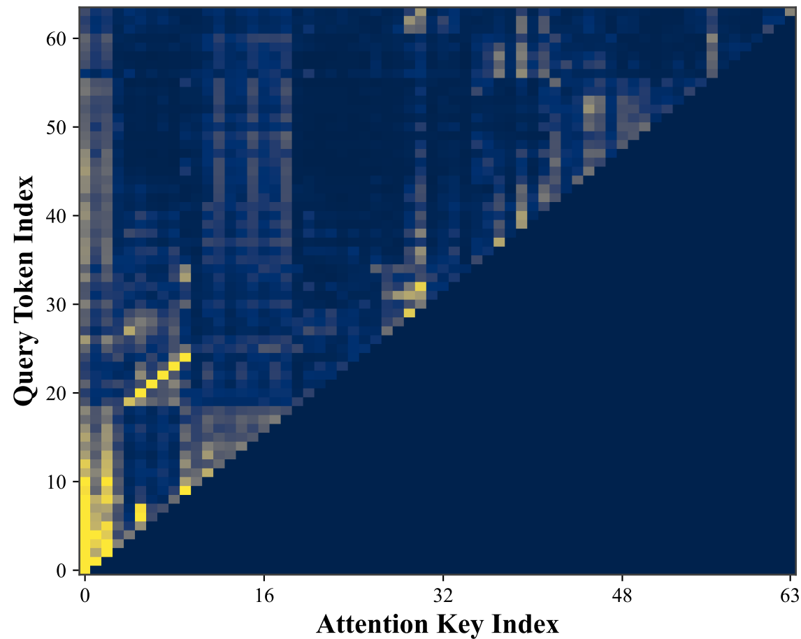
Row Tokens Baseline (Layer 13)
