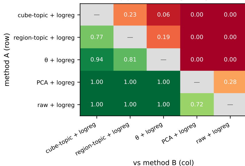
(d) HIDSAG — P[A > B]
