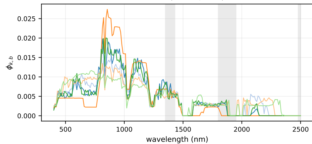
Kennedy Space Center (AVIRIS, K=12)
