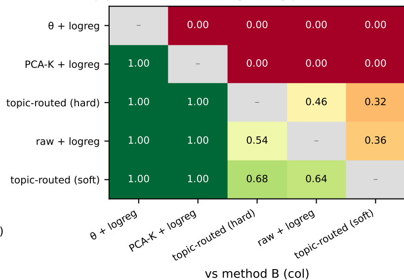
(d) HIDSAG: P[A > B] (hierarchical model)
