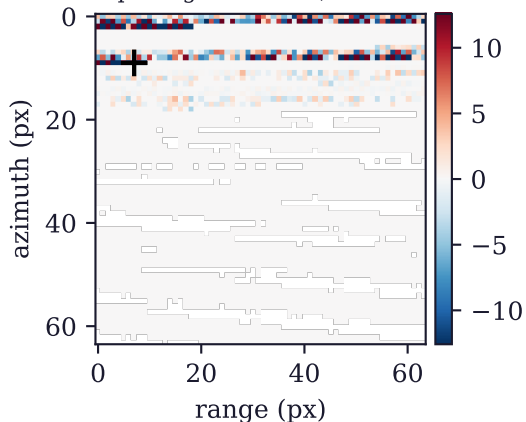
(a) LOS displacement map (mm) Campi Flegrei caldera, 2016-2018
