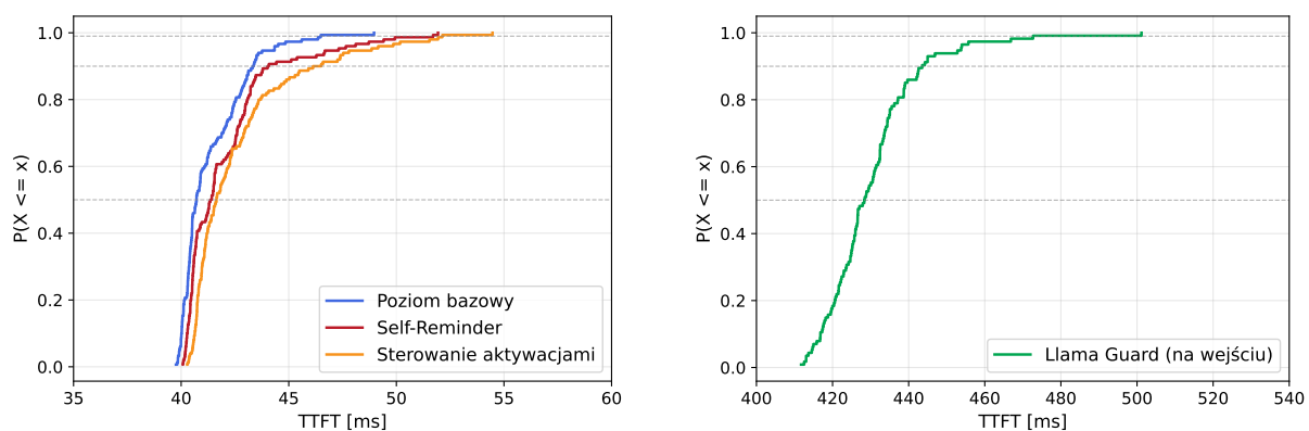
Rysunek 6. Porównanie dystrybuant empirycznych dla metryki TTFT dla metod obrony modelu Llama-3.1-8B-Instruct
