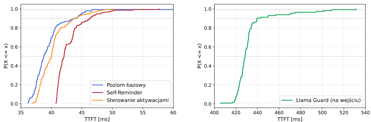
Rysunek 7. Porównanie dystrybuant empirycznych dla metryki TTFT dla metod obrony modelu Mistral-7B-Instruct-v0.3
