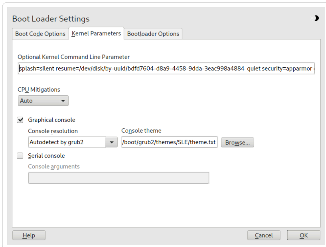
Figure 18.3.3.2.4. Kernel parameters
