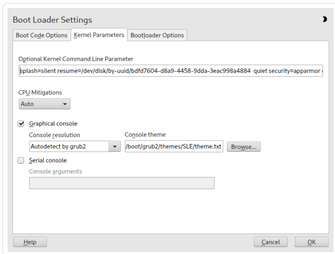
Figure 18.4. Kernel parameters
