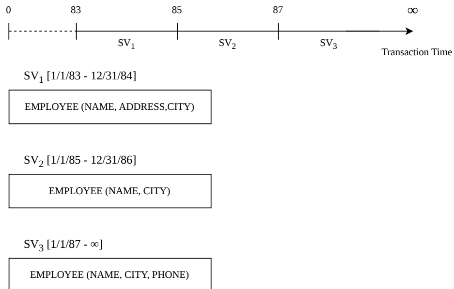
Abbildung 4: Transaktionszeitbasierte Schema-Versionierung
