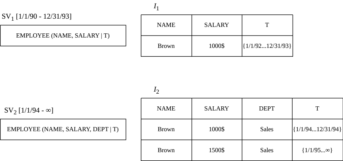
Abbildung 10: Synchrones Management
