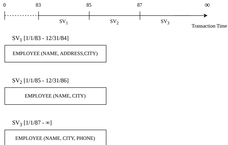
Abbildung 9: Transaktionszeitbasierte Schema-Versionierung
