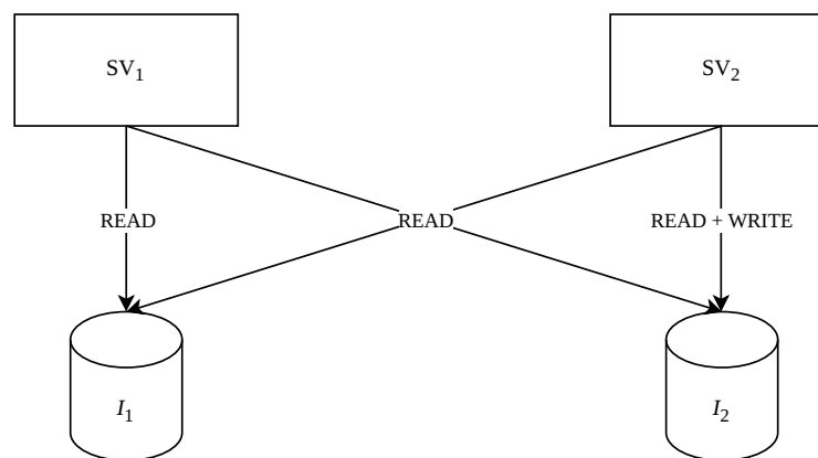
Abbildung 7: Partielle Schema-Versionierung
