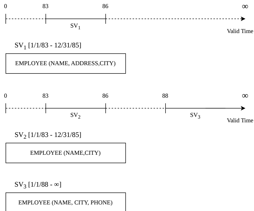
Abbildung 10: Gültigkeitszeitbasierte Schema-Versionierung
