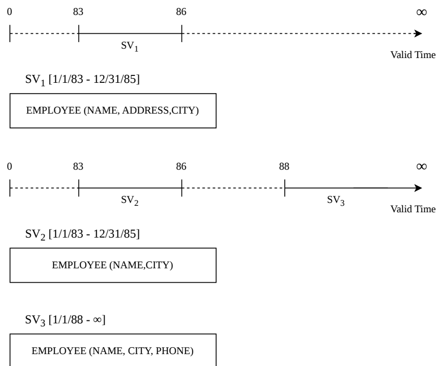
Abbildung 4: Gültigkeitszeitbasierte Schema-Versionierung
