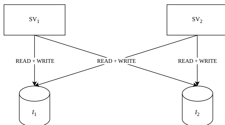
Abbildung 2: Vollständige Schema-Versionierung
