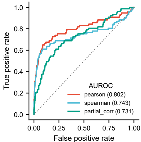
ROC · TF→target
