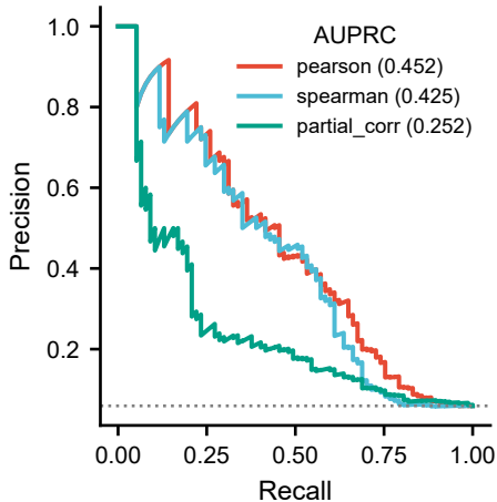
Precision-recall · TF→target
