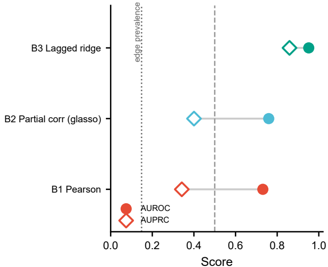
AUROC vs AUPRC
