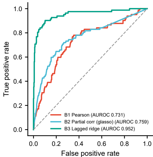
Edge recovery
