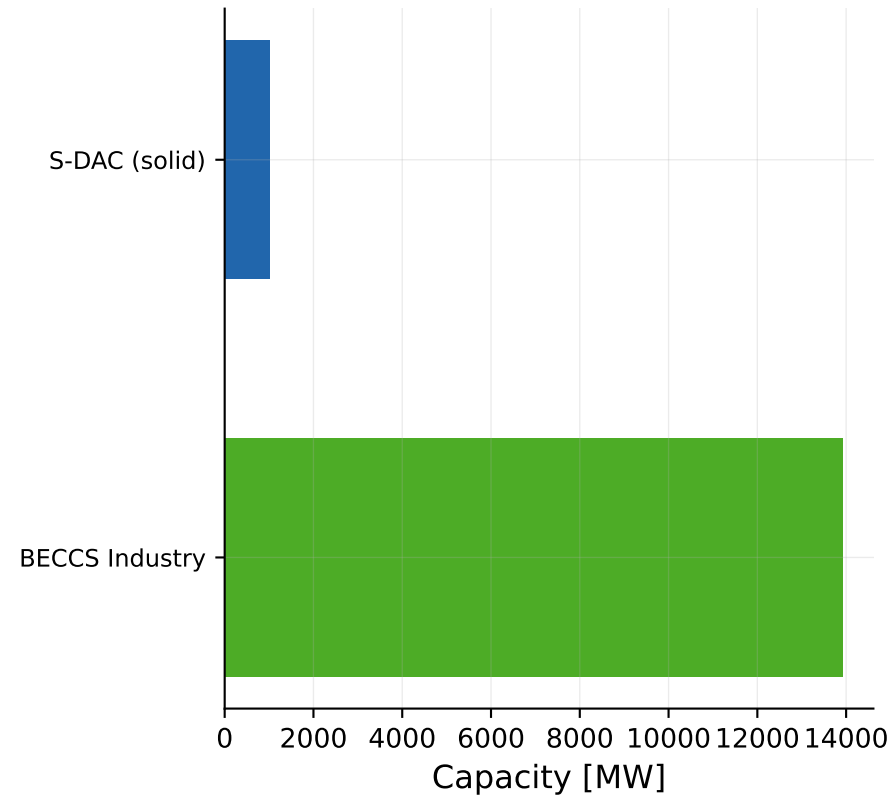
2030 (at 200 EUR/tCO 2 )
