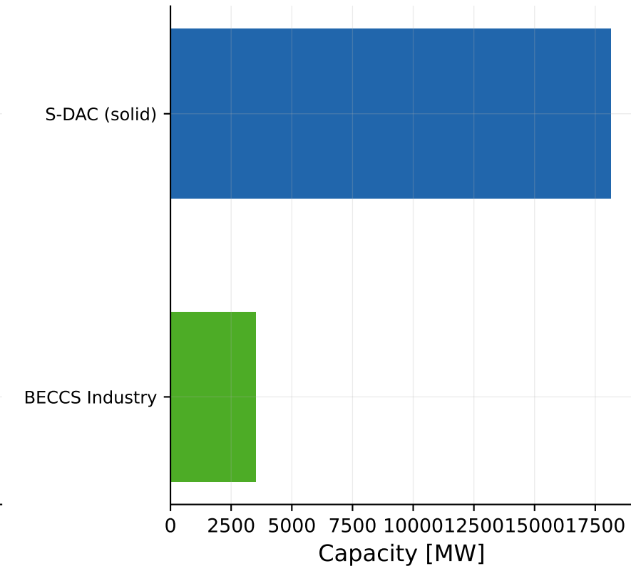
2050 (at 100 EUR/tCO 2 )
