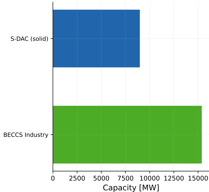
2040 (at 300 EUR/tCO 2 )
