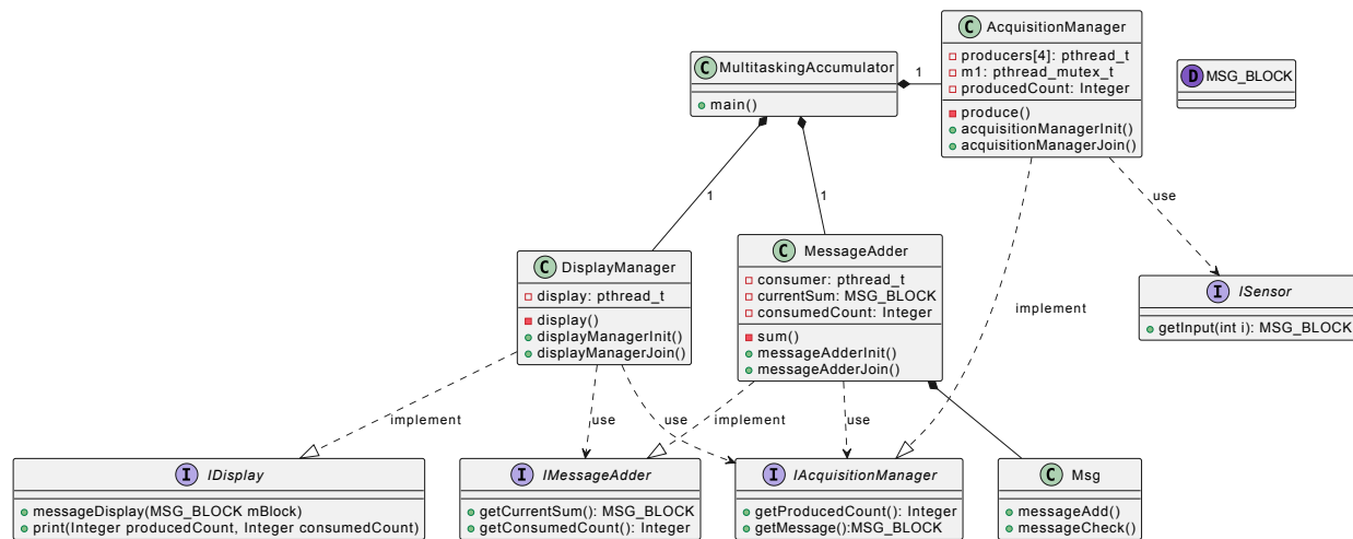
Figure 5: Architecture Logicielle Détaillée de MultitaskingAccumulator. La description de l'architecture logicielle détaillée mise en oeuvre.
