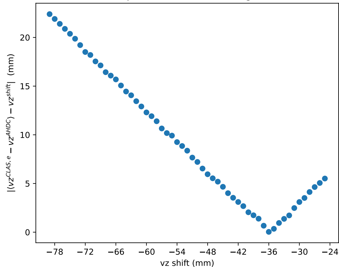
Optimal vz shift (inbending)
