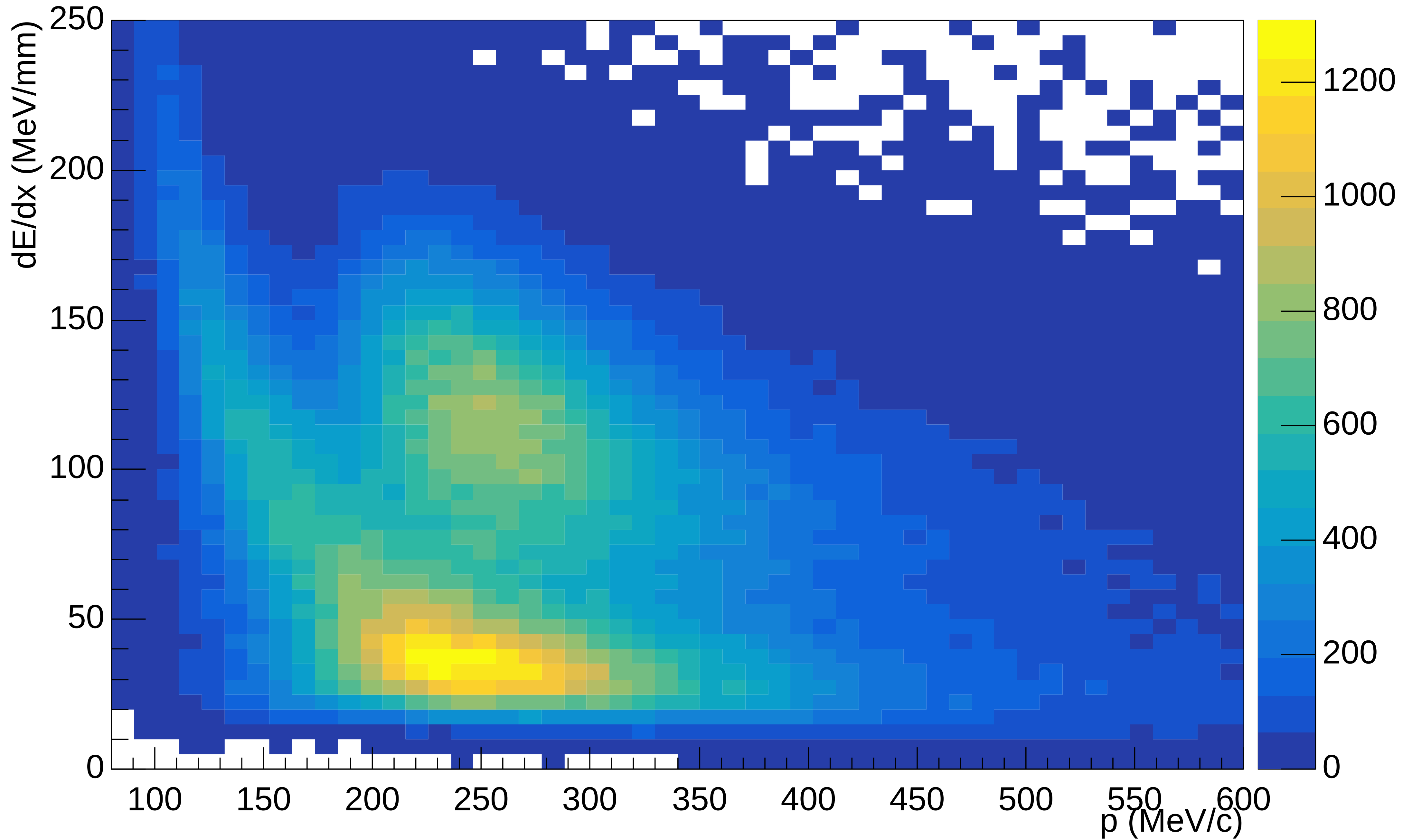
dE/dx vs p
