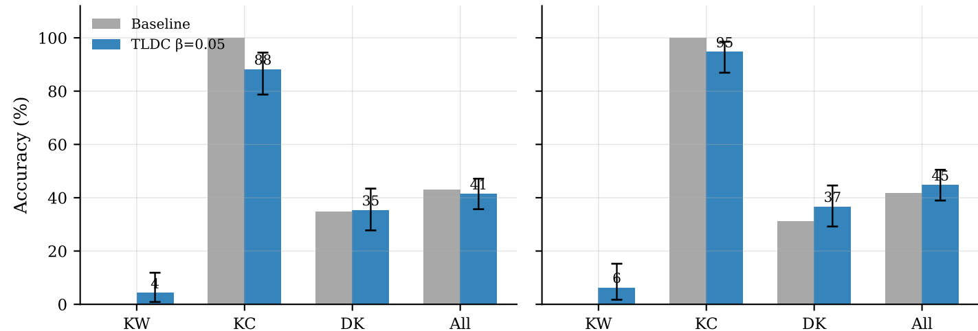
seed 123 (n=300)
