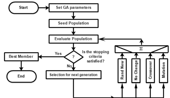
图5. 遗传算法流程图。
