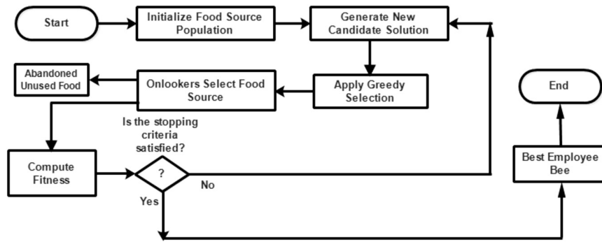
图 7. 人工蜂群算法流程图阶段。
