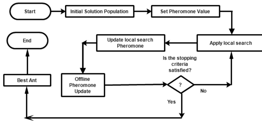
图 6. 蚁群优化搜索算法流程图
