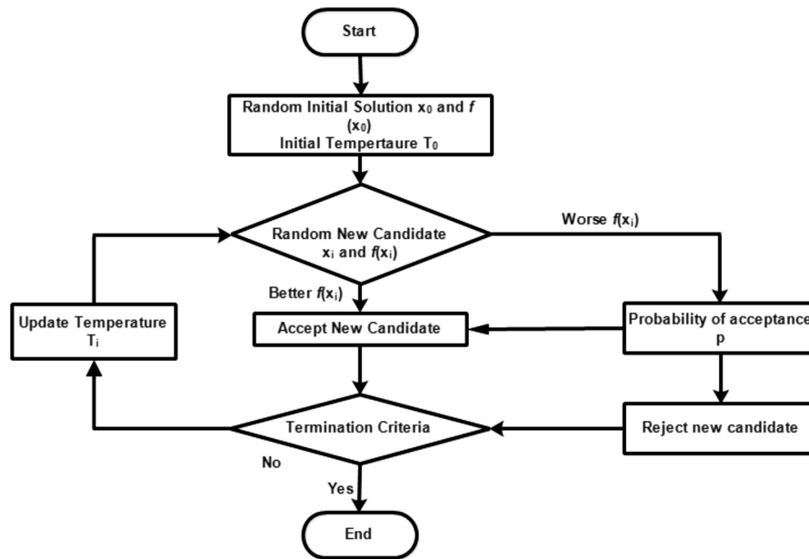
图 13.模拟退火算法流程图。
