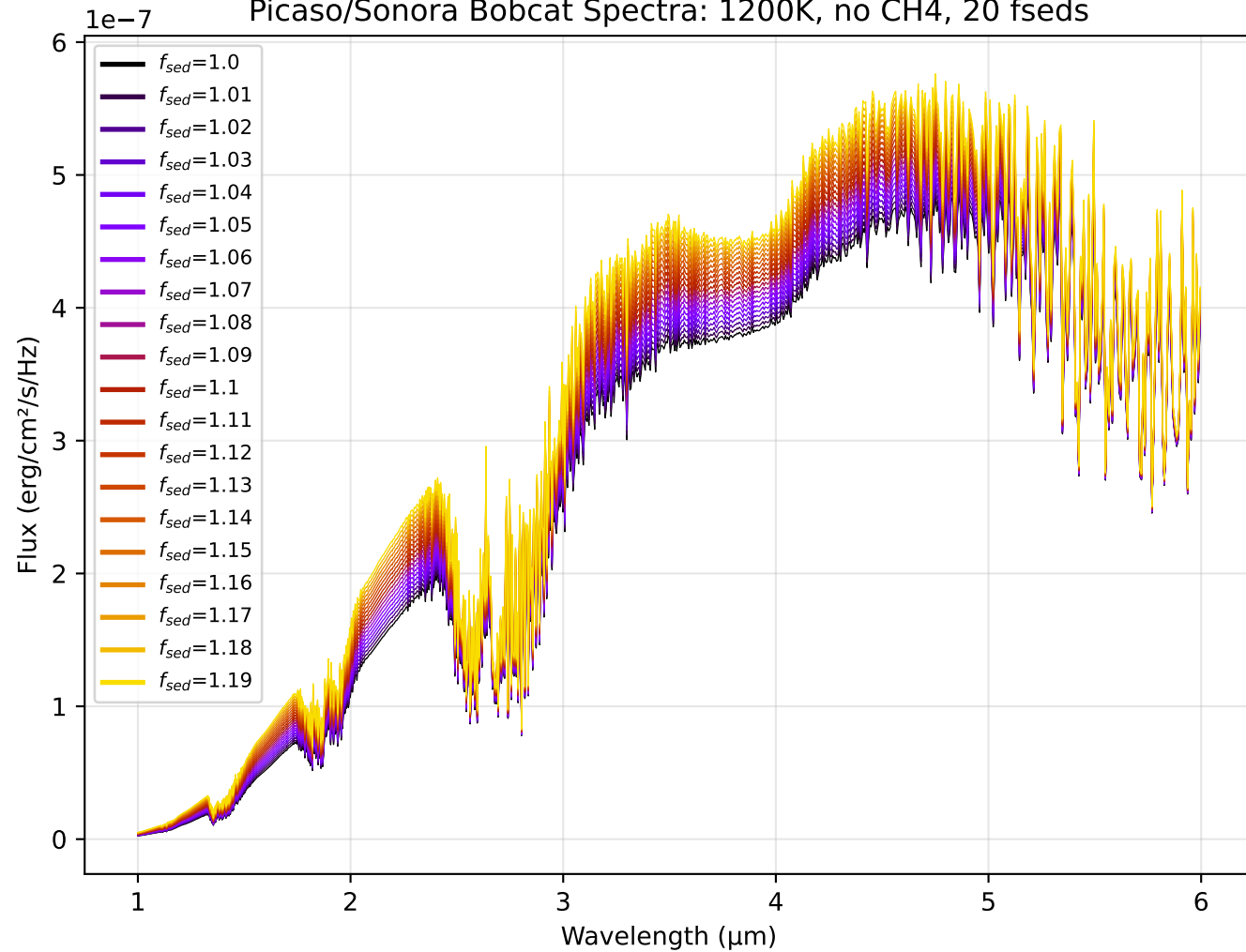
Picaso/Sonora Bobcat Spectra: 1200K, no CH4, 20 fseds
