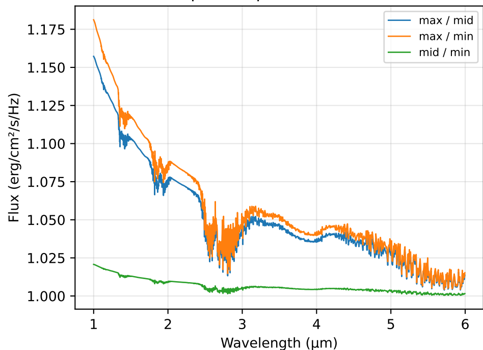
Composite Spectra Ratio; i=80
