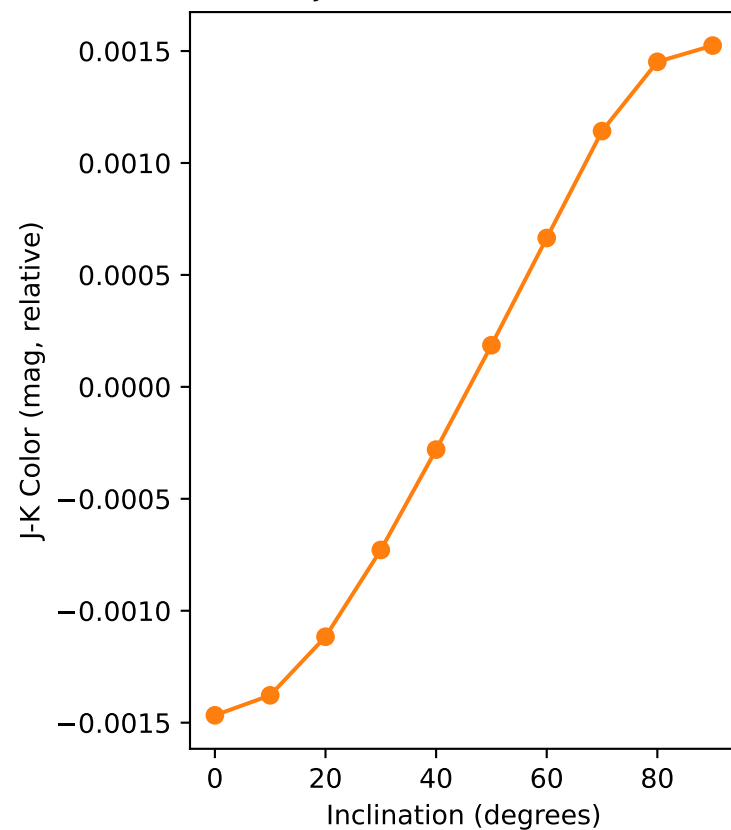
J-K Color vs Inclination
