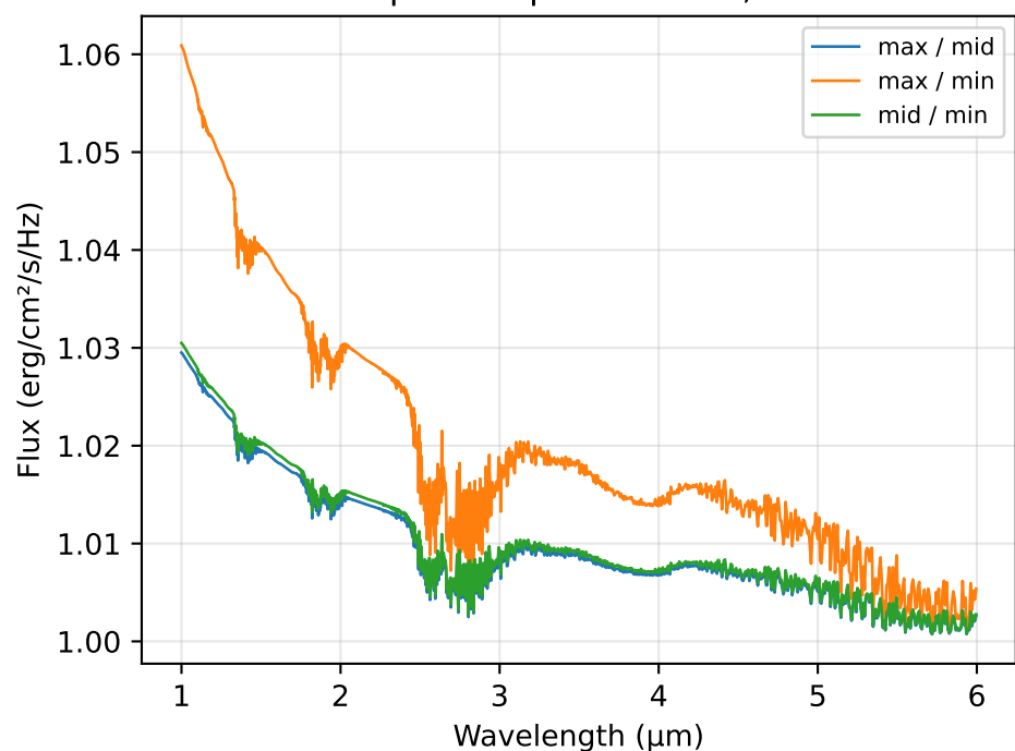
Composite Spectra Ratio; i=40
