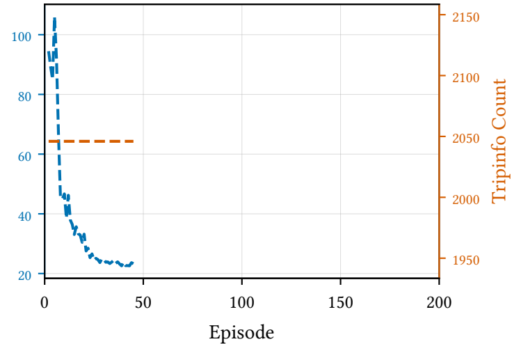
MLP+GATv2+SAC
