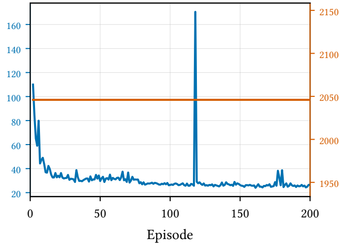
FRAP+GATv2+PPO
