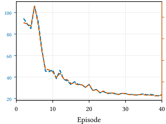
Cologne 8 SAC
