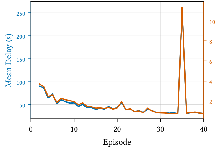
Cologne 8 PPO
