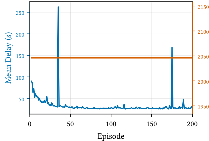
Cologne 8 PPO
