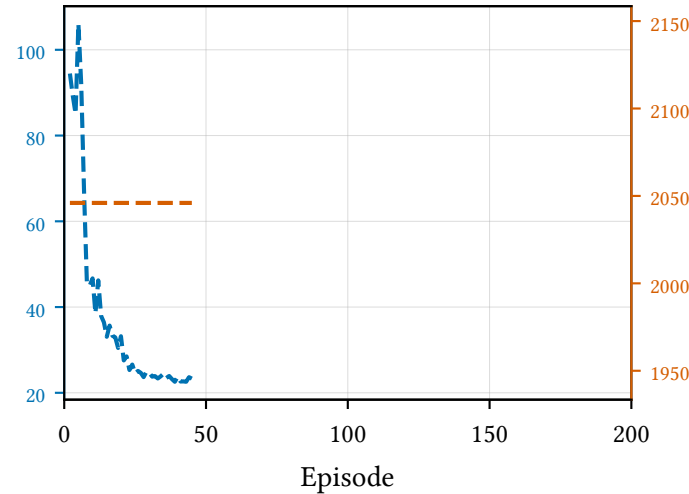
Cologne 8 SAC
