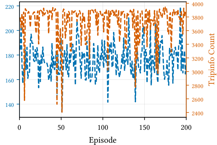
Ingolstadt 21 SAC
