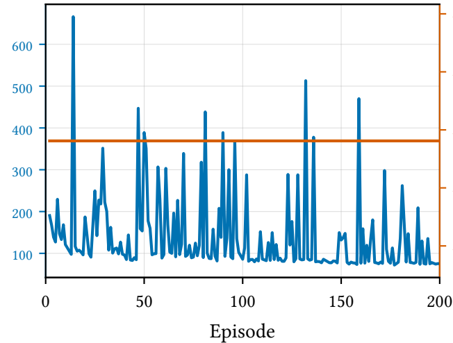
Ingolstadt 21 PPO
