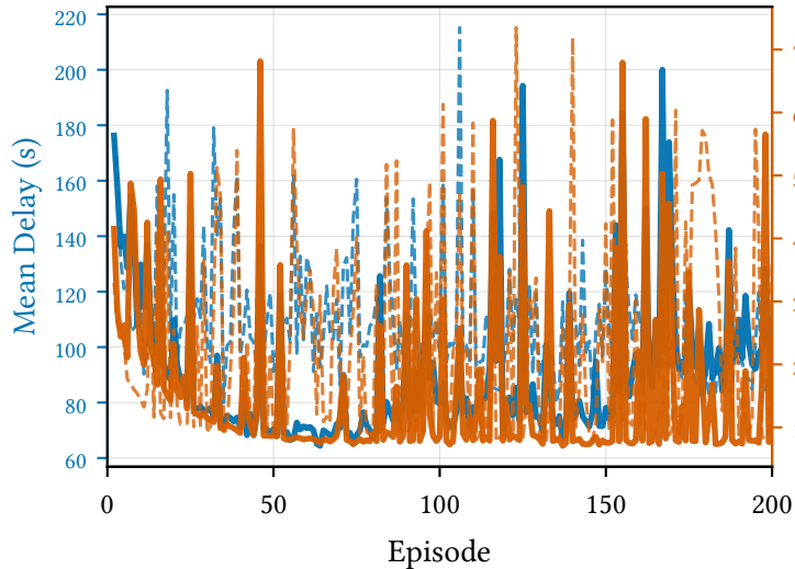
Ingolstadt 21 PPO
