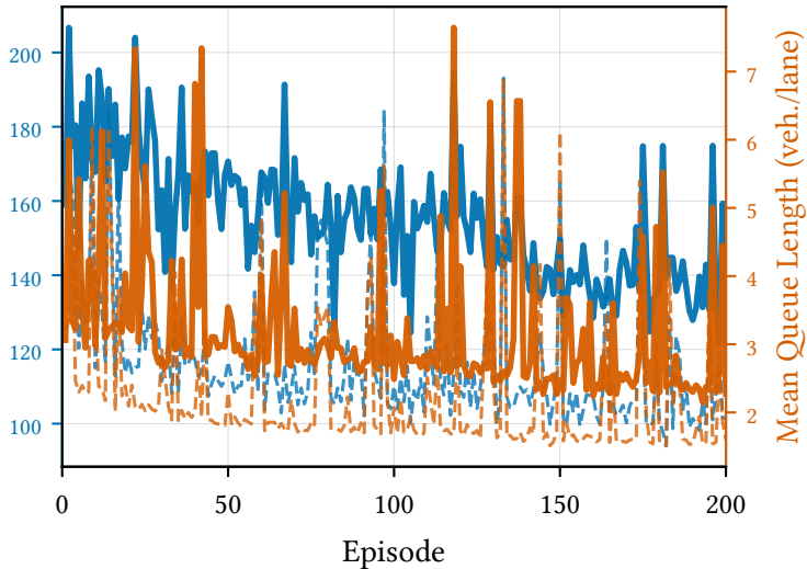
Ingolstadt 21 SAC
