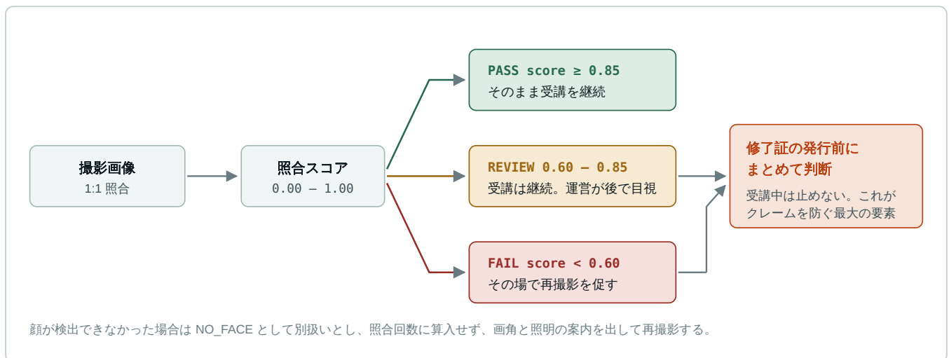
fig.2 - 3段階判定。REVIEW と FAIL のどちらでも、その場では受講を打ち切らない。
