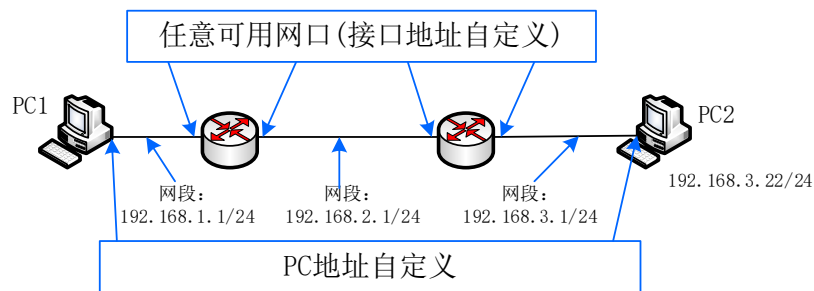
图 1 静态路由实验拓扑
