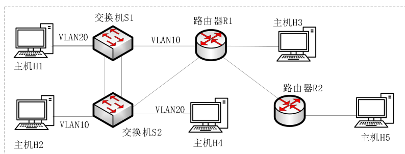
图 1. 实验拓扑
