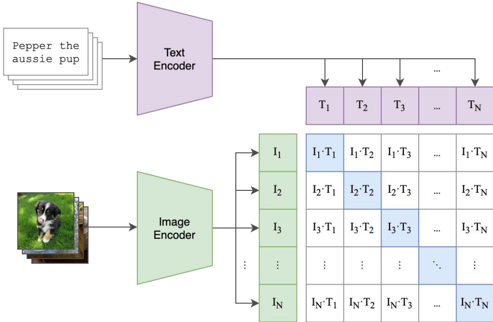
CLIP
