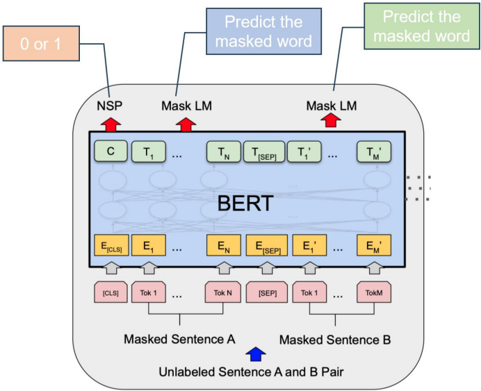
BERT
