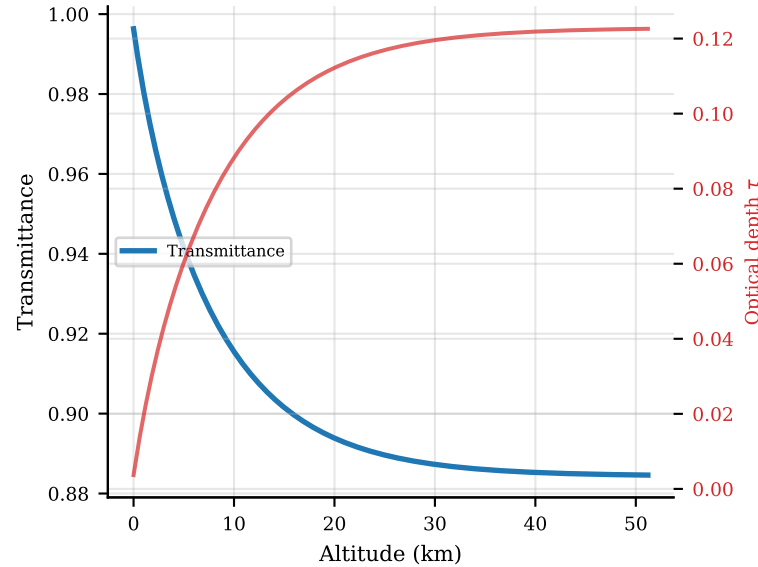
(D) Zenith transmittance
