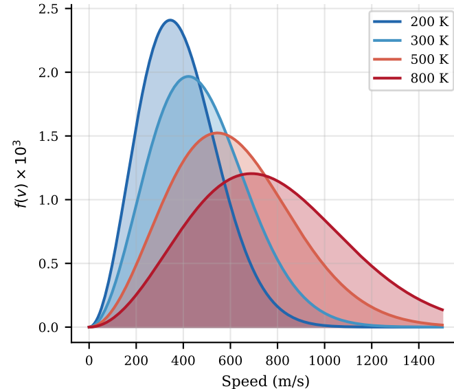
(D) Maxwell-Boltzmann ( N_2 )
