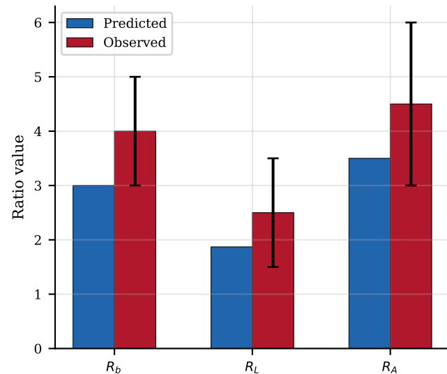
(D) Horton ratios
