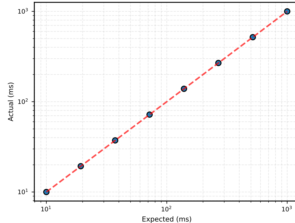
D. Spacing
