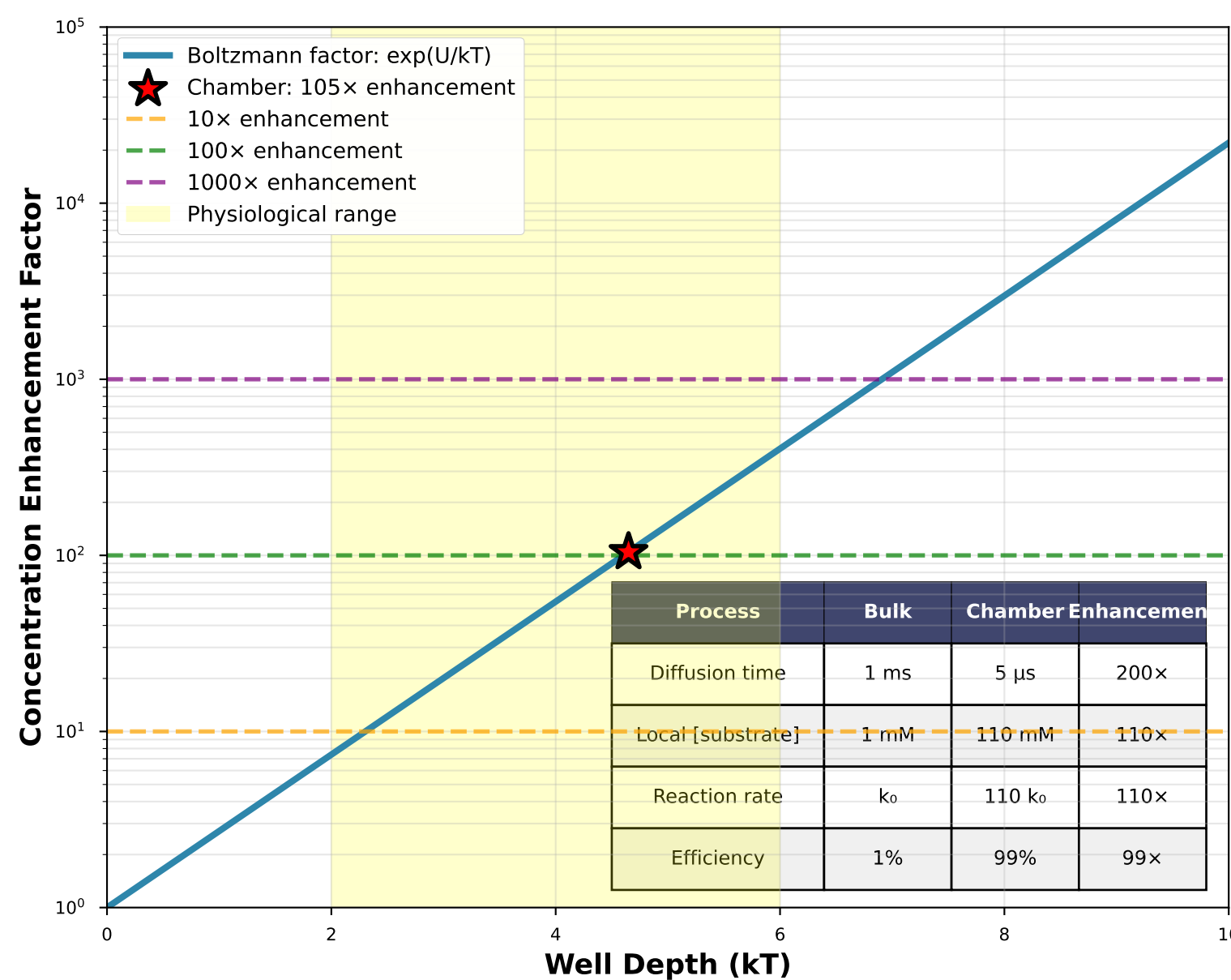
(D) Reaction Rate Enhancement in Chambers
